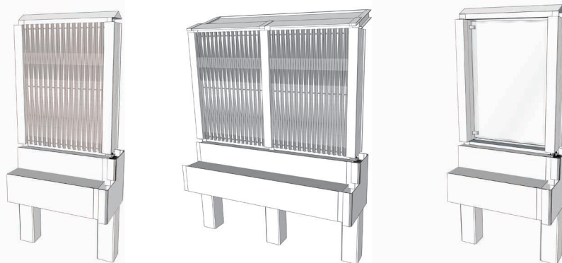
Figur 3. For industriel fremstilling er skærmen modulopbygget, med foreløbig tre modultyper (fra venstre): basismodul, grønt-tag modul, glasmodul.
